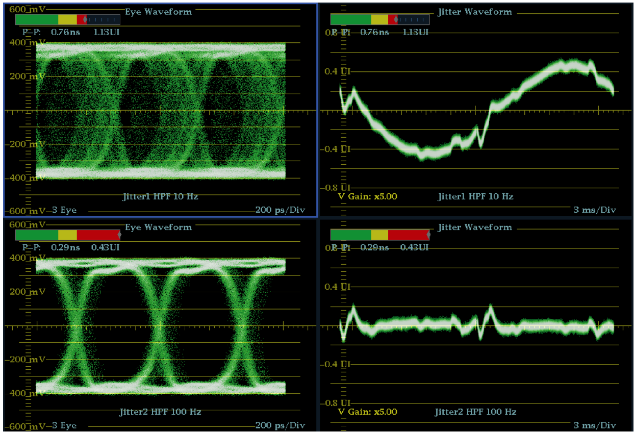
图 3： 测量抖动
